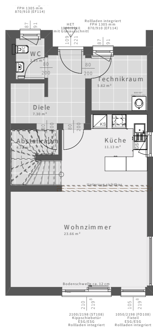
ERDGESCHOSS
